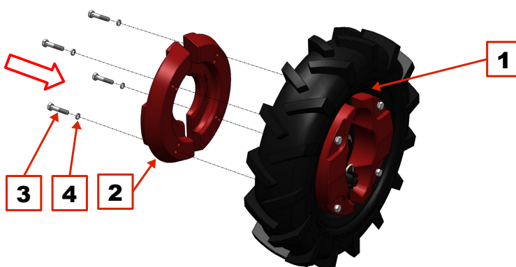
Montáž závaží a šroubů s podložkami
