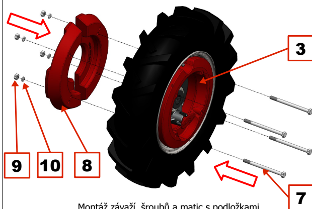
Montáž závaží, šroubů a matic s podložkami
