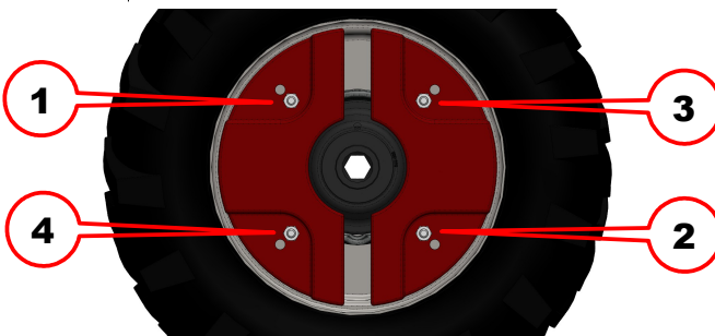
Montáž závaží, šroubů a matic s podložkami
