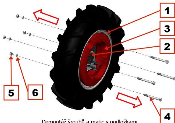
Demontáž šroubů a matic s podložkami
